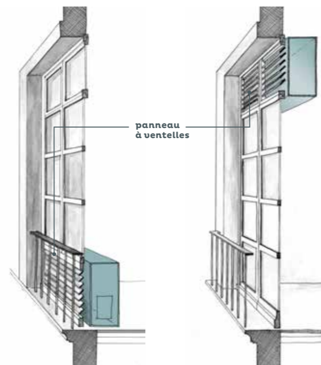
Exemple de grilles de ventilation intégrées dans les menuiseries
