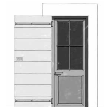
Porte extérieure vitrée avec petits bois, panneau mouluré en partie basse et volet de protection à doubles lames de bois croisées
